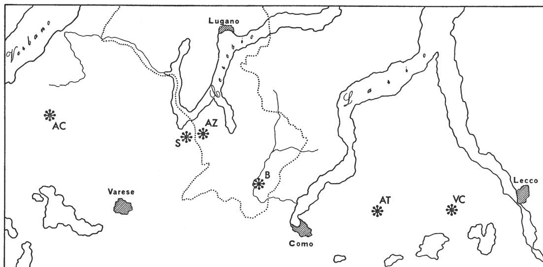
Fig. 1 - Localizzazione delle serie considerate - AC: Arcumeggia; S: Saltrio; AZ: Arzo, cava del cimitero; B: Breggia; AT: Alpe Turati; VC: Val Cappelletto.
