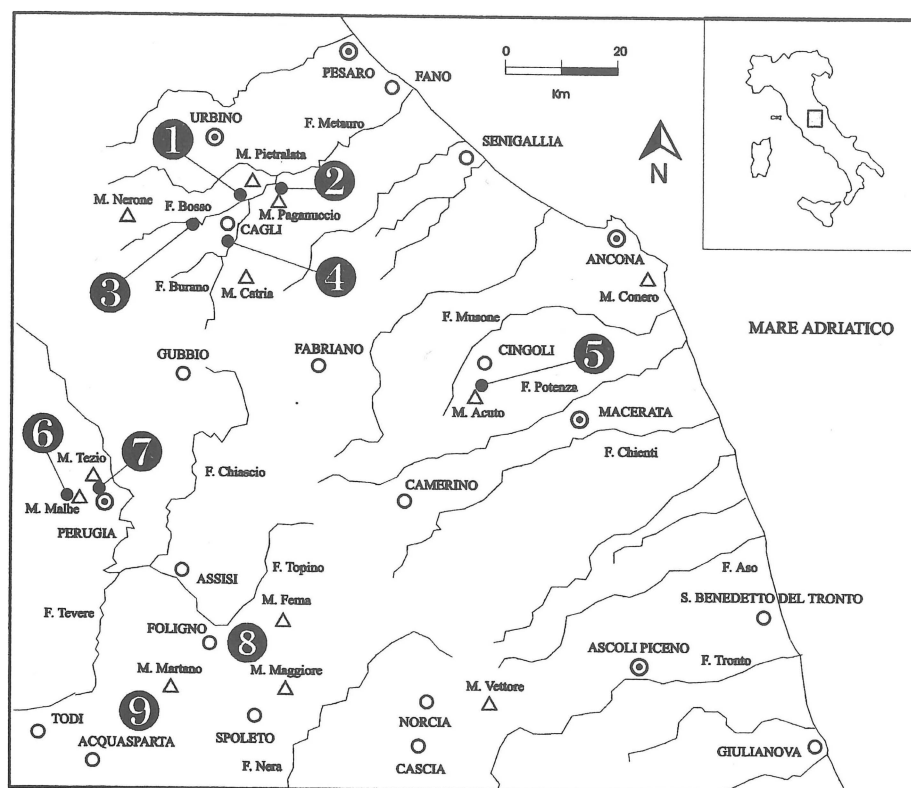
Text-fig. 1 - Location of the stratigraphic sections studied. 1) P.so del Furlo, Grilli Quarry CG; 2) P.so del Furlo, S. Anna Quarry SA; 3) F. Bosso, "Eremita" section, B.ER and "I Lecceti" section, Le; 4) F. Burano, Bu; 5) Cingoli, S.I.E.L.P.A. Quarry, SIE; 6) Migiana di M. Malbe, MM; 7) F.so della Colognola-M. Tezio, FCT; 8) M. di Civitella, MC and Pettino, Pe; 9) Cima Panco, CP and F.so di Pozzale, Po.
